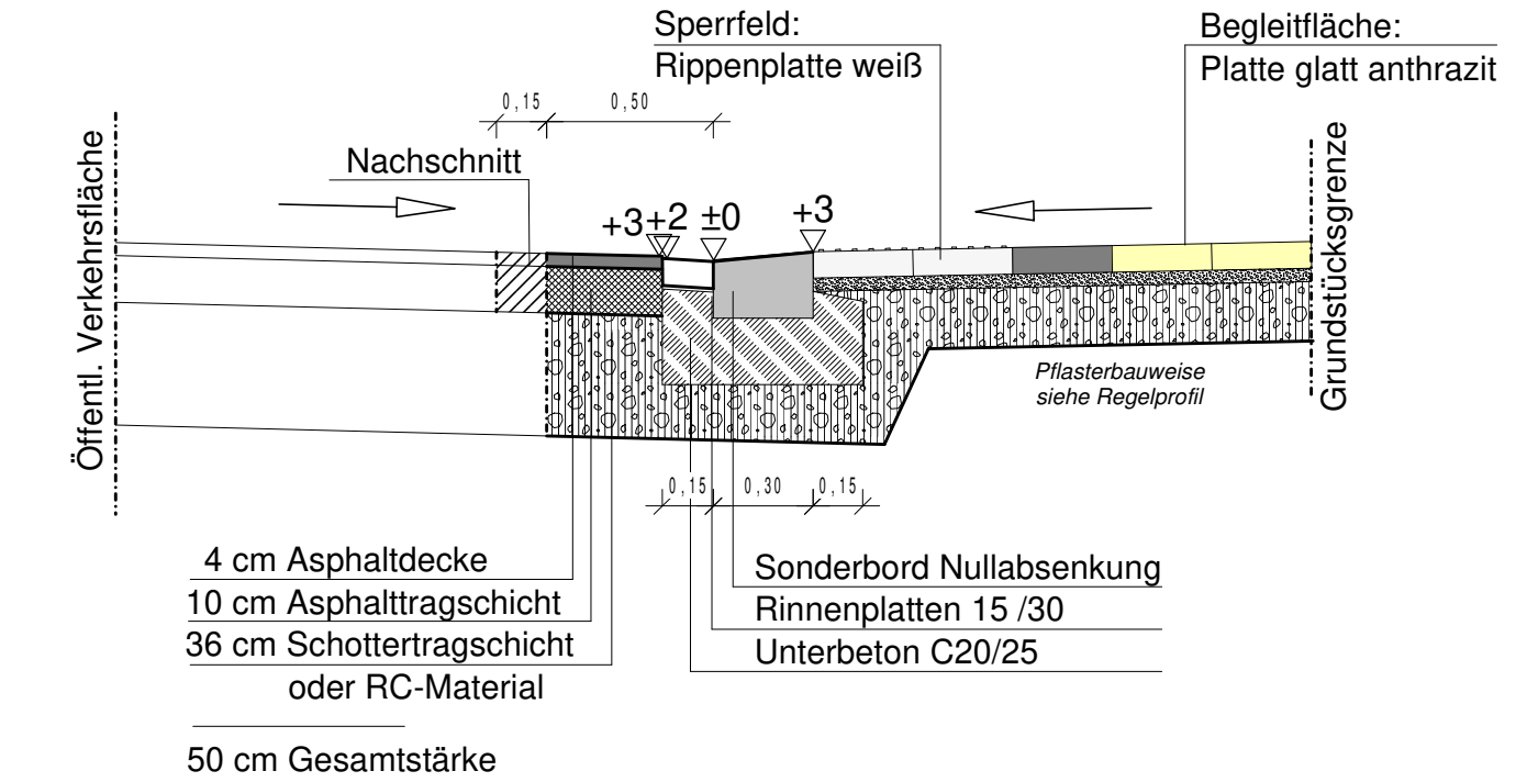
Detail A-A M 1 : 25
