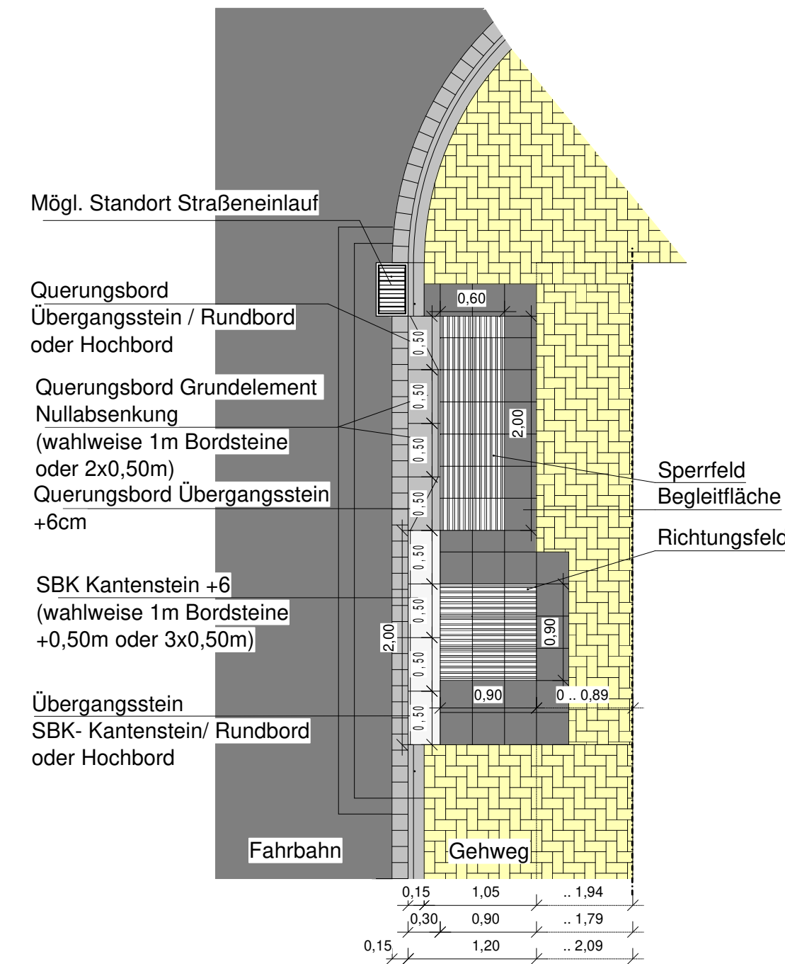
Detail Ungesicherte Querungsstelle 1,20m - 2,09m
