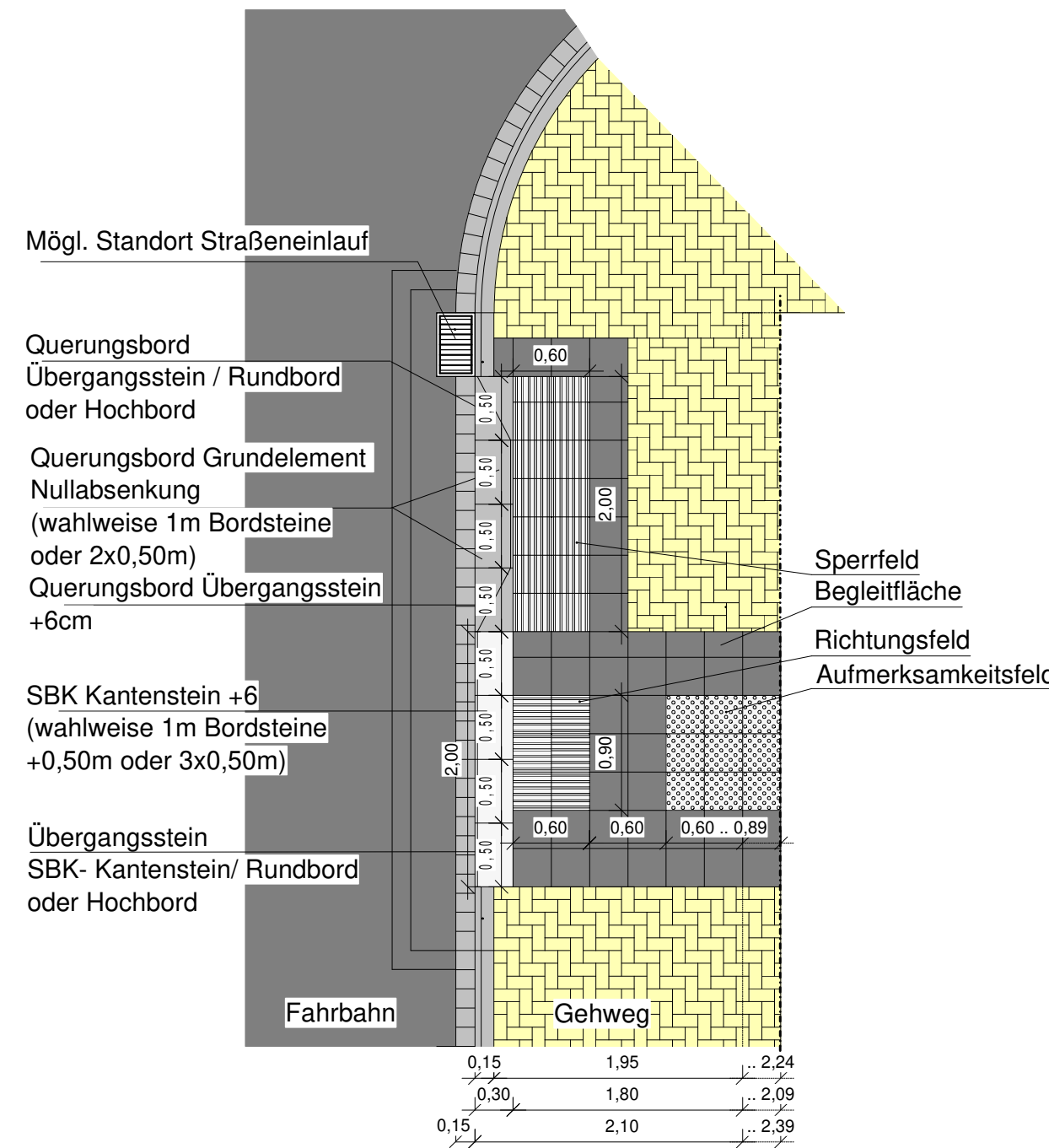
Detail Ungesicherte Querungsstelle 2,10m - 2,39m
