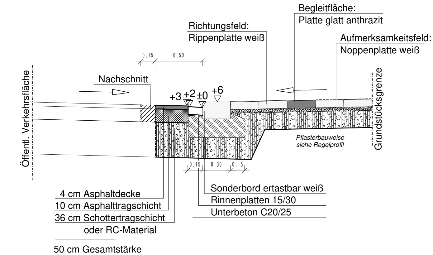
Detail B-B M 1 : 25
