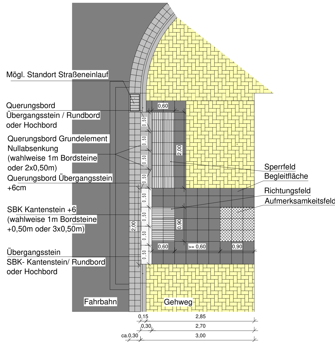
Detail Ungesicherte Querungsstelle >=2,40m (z. B. 3,00m)
